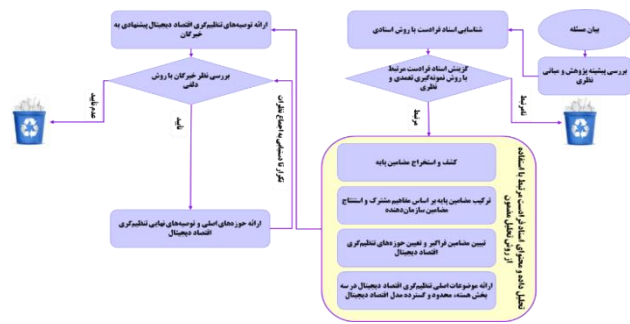
شکل ۲- مراحل پژوهش
